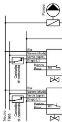
COLLEGAMENTO DEL FERMO POMPA CON DUE SERVOCOMANDI 2 PUNTI CONNECTION OF THE PUMP STOP WITH TWO 2-POINT ACTUATORS
