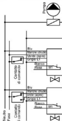
COLLEGAMENTO DEL FERMO POMPA CON UN SERVOCOMANDO 3 PUNTI ED UNO 2 PUNTI CONNECTION OF THE PUMP STOP WITH ONE 3-POINT AND ONE 2-POINT ACTUATORS
