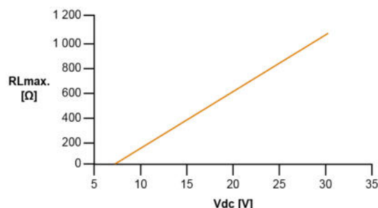
Résistance de charge par rapport à l'alimentation
