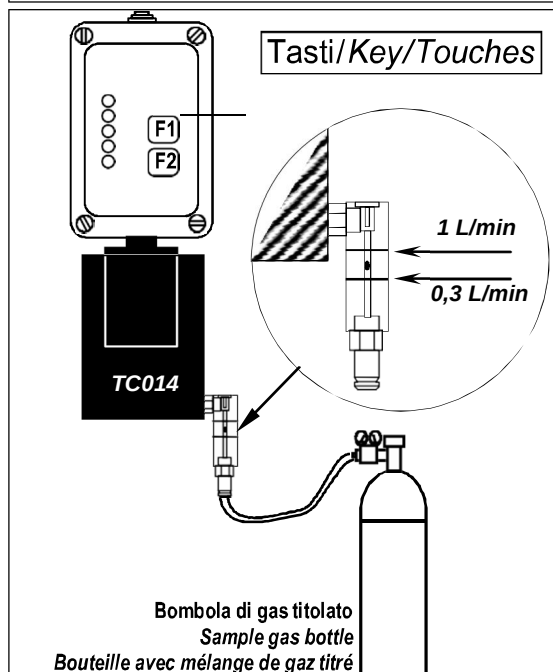
Fig. 3 - Tester di calibrazione/Calibration Tester/Kit de Calibration
