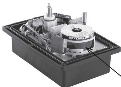
Résistance anti-condensation
