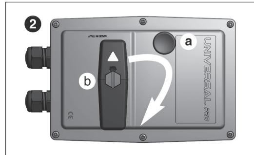
Servomoteur en position de fermeture
