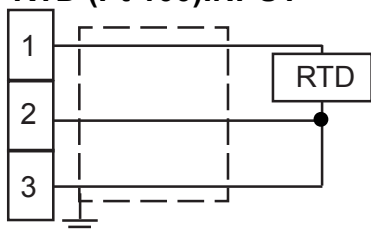
Fig. 5- RTD input wiring
