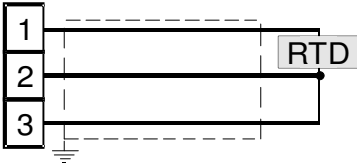
Fig. 5 Connexion de thermorésistance
