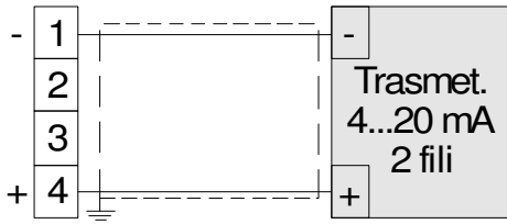
Fig. 8 Connexion de signaux 0/4-20 mA à transmetteur passif avec alimentation auxiliaire
