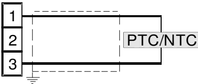
Fig. 6 Connexion de thermisteur
